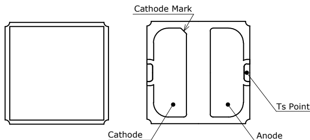
図2 T_s 測定ポイント (NCSU434x)
