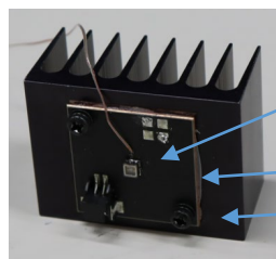
写真 2 評価した光源の構成 (NCSU434x)
