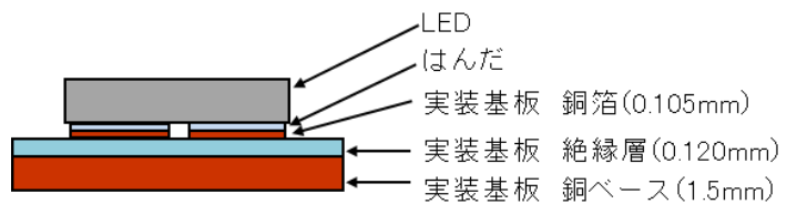
図 3 実装構造
