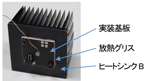
写真 3 評価した光源の構成 (NCSU434x)
